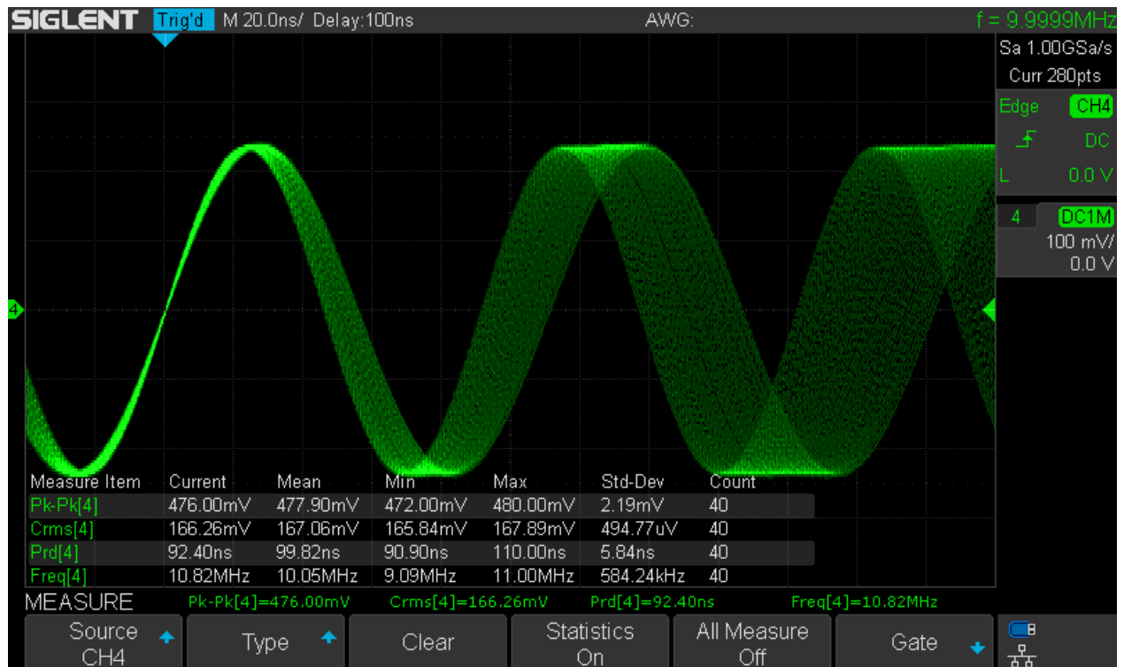
Sine_10MHz_FM1kHz_D1MHz_M20ns_Dots
